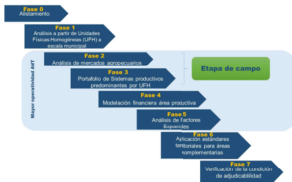
Figura 7. Flujograma del proceso metodológico para el cálculo de la UAF
