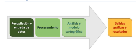
Figura 15. Proceso de análisis de información espacial para la obtención del mapa de las unidades físicas homogéneas
