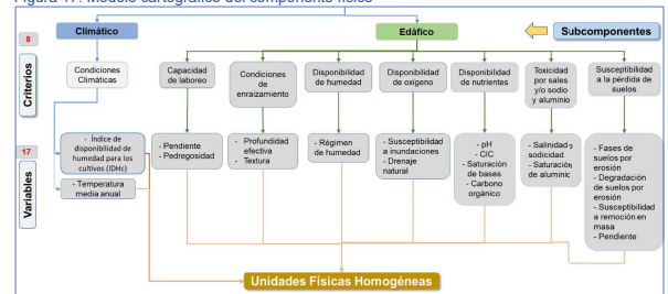
Figura 17. Modelo cartográfico del componente físico
